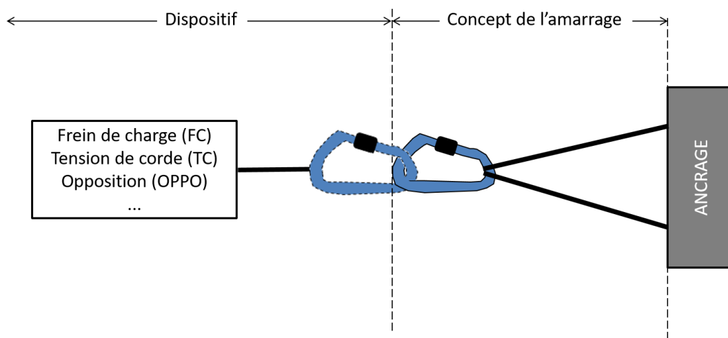
Conversion d'un dispositif. © Nicolas Comes - DGSCGC
