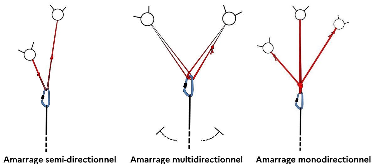
Exemples de répartition avec une charge. © Nicolas Comes - DGSCGC
